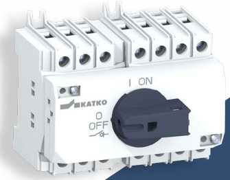
KU 640NO kiinteän NO (normal open) apukoskettimen kanssa (KU 340 kytkin + KU 340NO kytkin + PK40KU3P rinnakkaisvivusto)
