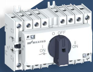
KU 340CO vaihtokytkin (1-0-2) ja kaksi apukosketinta (1NO40KU) molemmilla sivuilla
